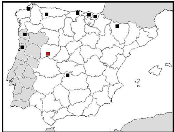
Mapa 1. Distribución ibérica de la especie. En rojo el registro objeto de esta nota, en negro los previos publicados.
